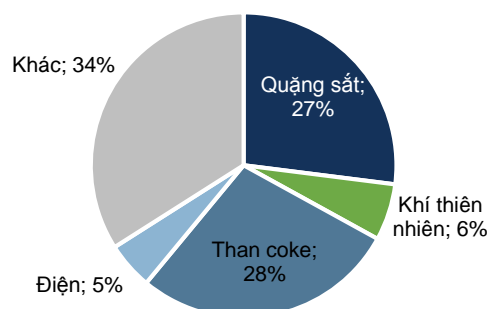
Cơ cấu chi phí luyện thép bằng lò BOF
